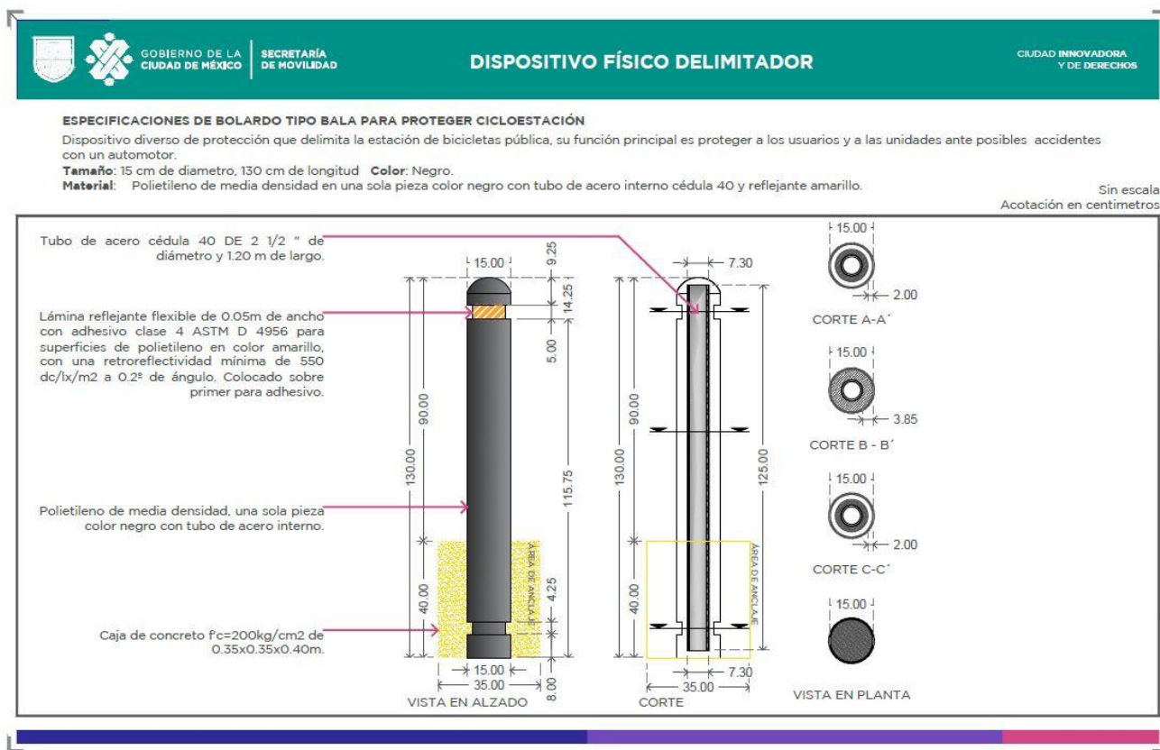
Figura 1. Bolardo tipo bala (cicloestación actual)
