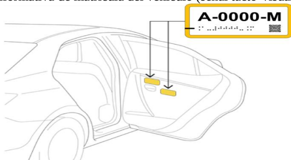
Esquema 10. Opciones de ubicación de placa informativa de la matrícula del vehículo en formato accesible visual y táctil en puerta trasera.
