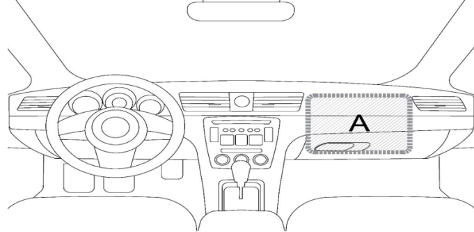
Esquema 7. Espacio donde debe ser colocado el rótulo de matrícula interior en la parte frontal del tablero del lado derecho, zona "A". El rótulo debe quedar de frente al usuario para garantizar su legibilidad.
