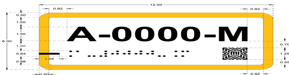
Esquema 9. Placa informativa de matrícula del vehículo (señal tacto-visual con sistema Braille).
