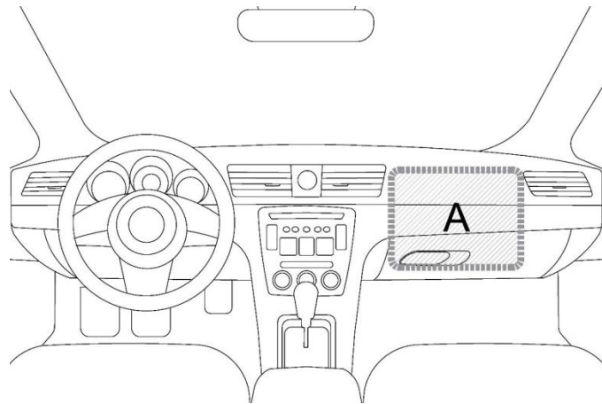
Esquema 7. Espacio donde debe ser colocado el rótulo de matrícula interior en la parte frontal del tablero del lado derecho, zona "A". El rótulo debe quedar de frente al usuario para garantizar su legibilidad.
