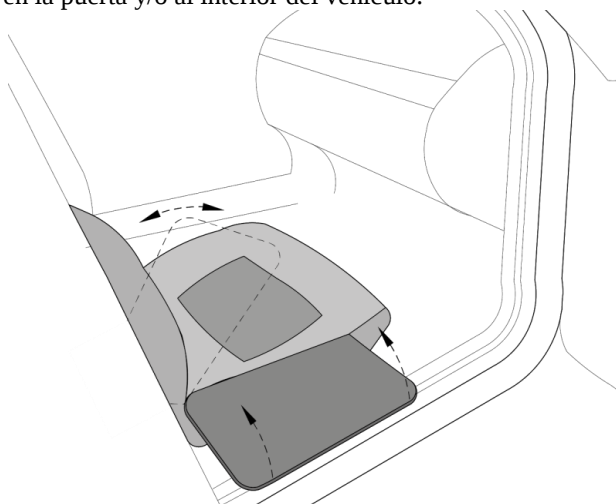
Esquema 11. Ejemplo de tabla de transferencia abatible y plegable para facilitar la transferencia, vista lateral.
