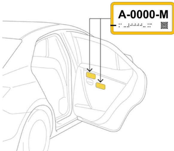
Esquema 10. Opciones de ubicación de placa informativa de la matrícula del vehículo en formato accesible visual y táctil en puerta trasera.
