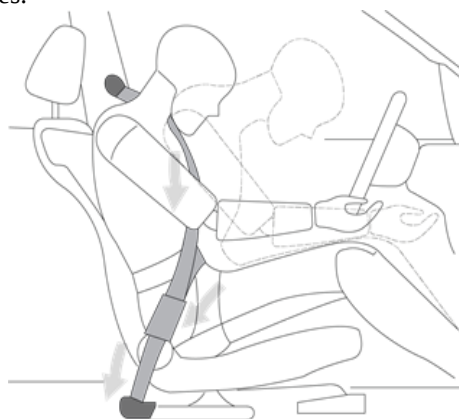
Esquema 4. Vista de reposacabezas y cinturón de seguridad
